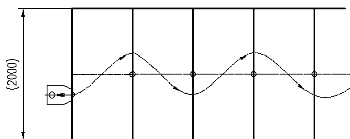
图 2 无碳小车在重力势能作用下自动行走（S 赛道）示意图
